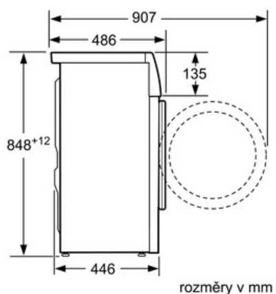
Rozměrové výkresy
