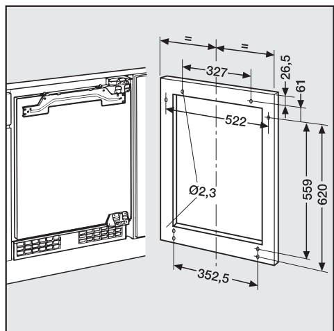
Obrazec vrtání v kazetových dvířkách
